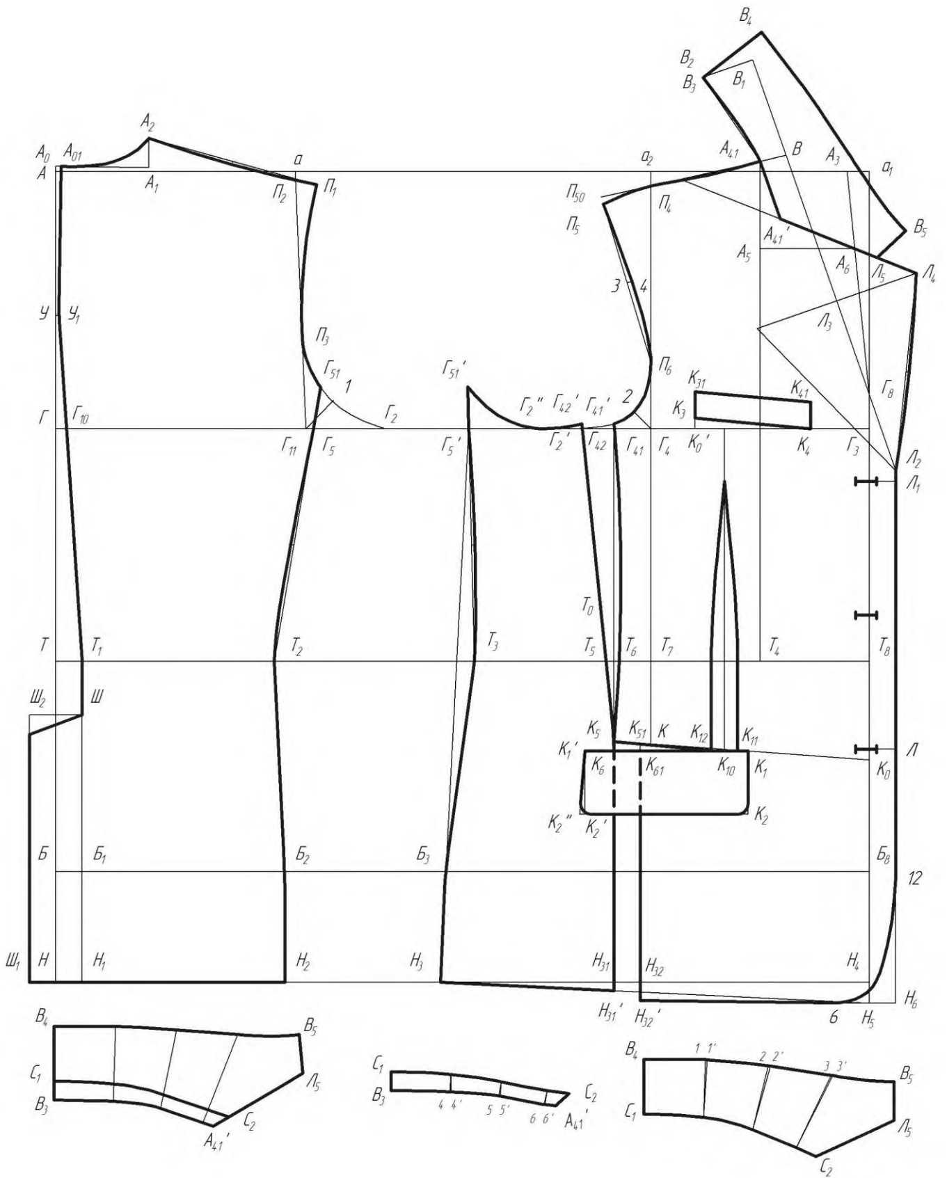
Рисунок 4. Чертёж модельной конструкции мужского пиджака
