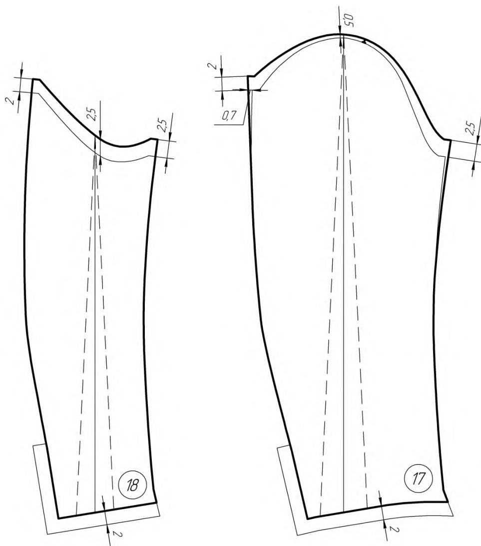
Рисунок 10. Производные лекала из подкладочной ткани мужского пиджака: верхняя и нижняя части рукава мужского пиджака
